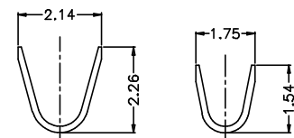
A-A SECTION
