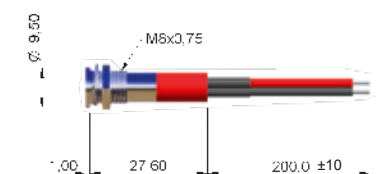
WIRES
