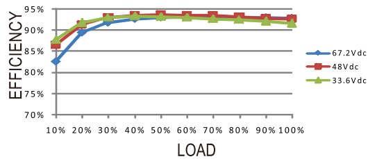
DDR-240C-24
