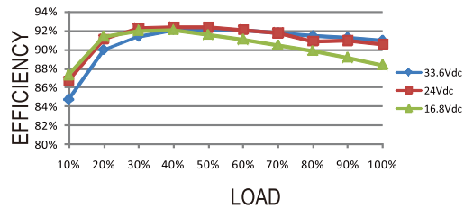
DDR-240B-24
