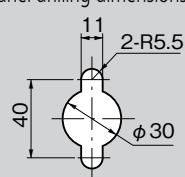
パネル穴明け寸法 Panel drilling dimensions
