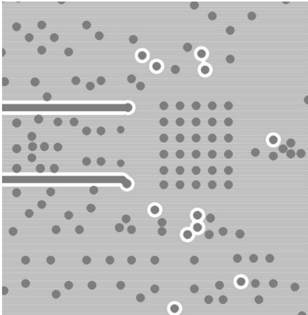
Inner Layer 4
