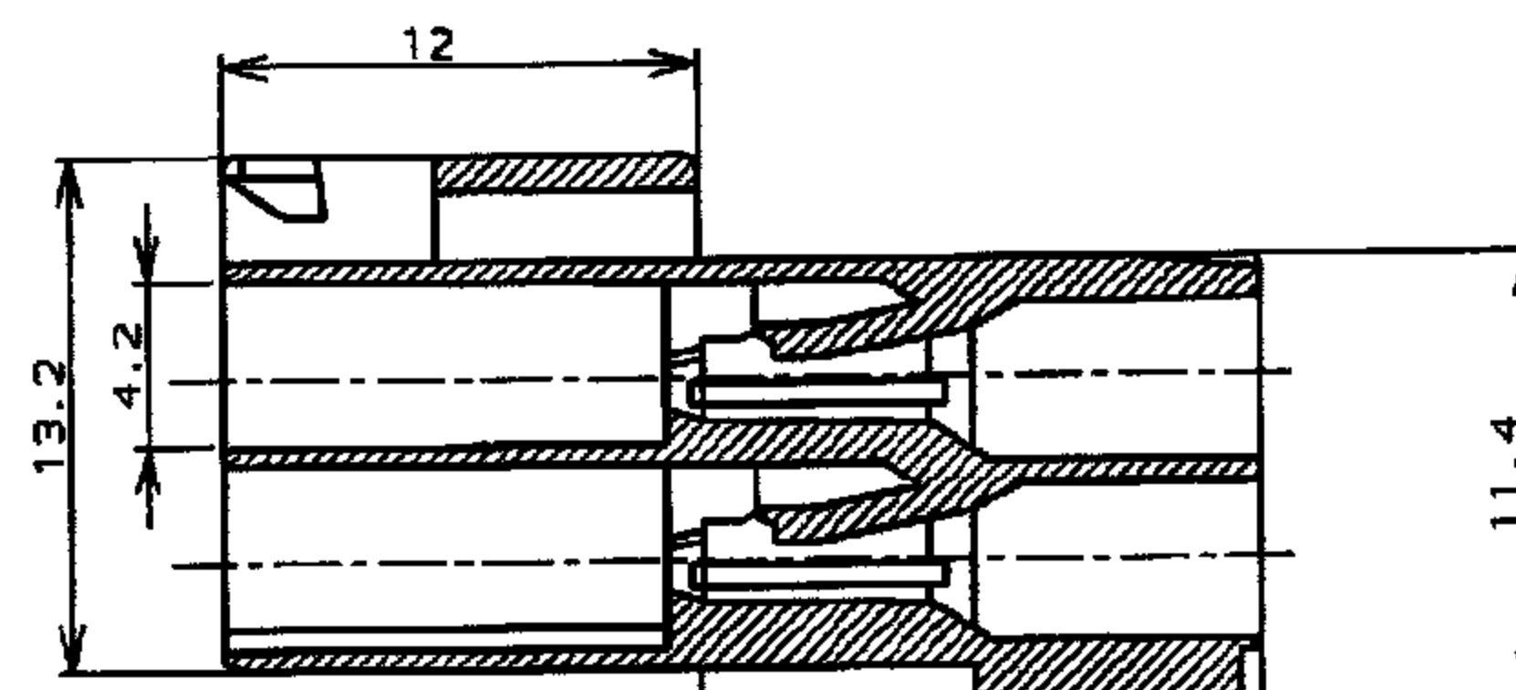
断面 "A-A" (SECT)
