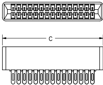
-- C -- DREN
