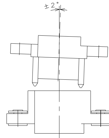
ALLOWABLE MATING ANGLE 傾き嵌合許容角度
