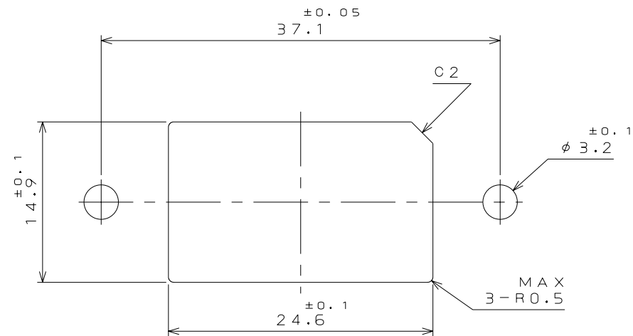
MOUNTING PANEL CUTOUT DIMENSIONS (REF.) パネル取付穴寸法 (参考)
