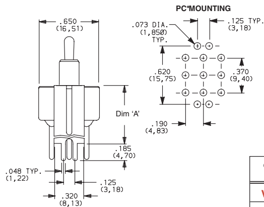
7301MD9__BE 3PDT
