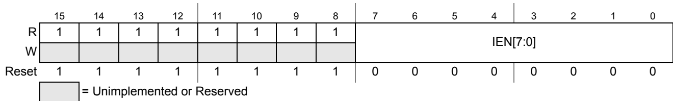
Figure 11-12. ATD Input Enable Register (ATDDIEN)
