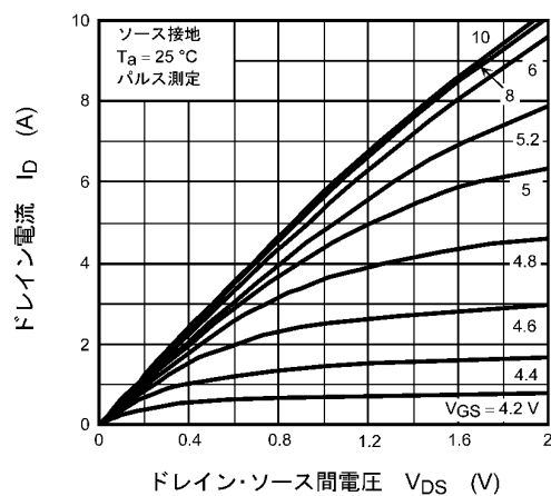
図 8.2 I_D - V_{DS}
