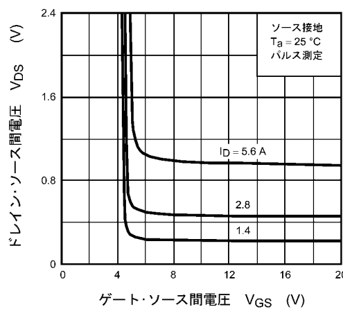
図 8.4 V_{DS} - V_{GS}
