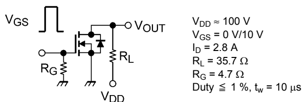
図 6.2.1 スwitchング時間の測定回路例
