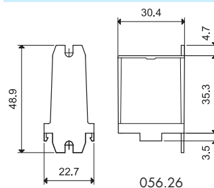
Top 35 mm rail (EN 60715) adaptor for 55.32, 55.33, 55.34
