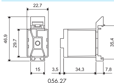
Top 35 mm rail (EN 60715) adaptor for 55.32, 55.33, 55.34
