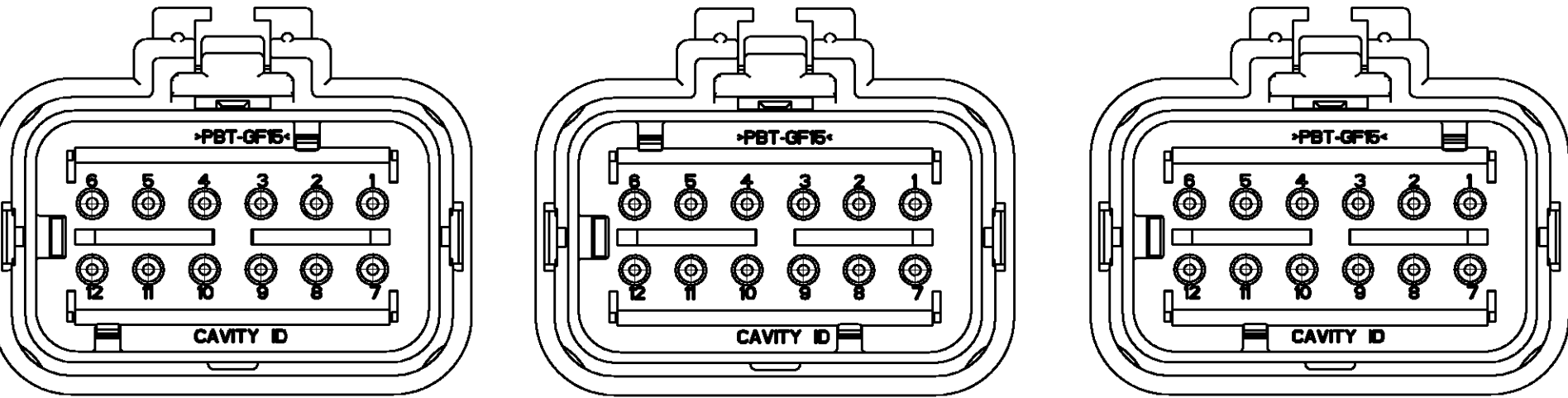
776533-2 SCALE 2:1
