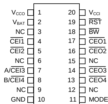
DS1323E 20-Pin TSSOP (173 mils)
