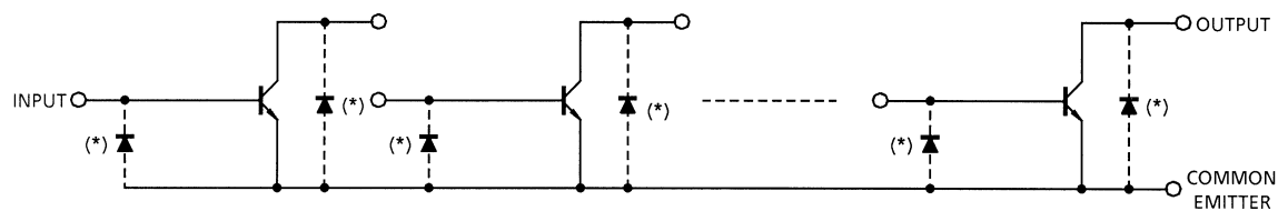
TD62502P / F
