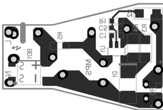
Bottom Layer
