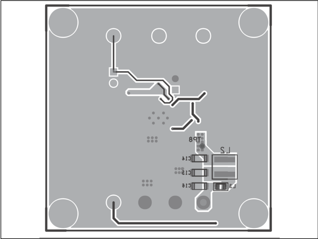
Figure 56. Bottom layer
