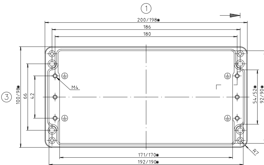
Unterteil
