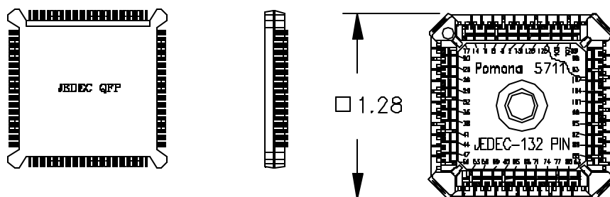
132 PIN JEDEC CHIP
