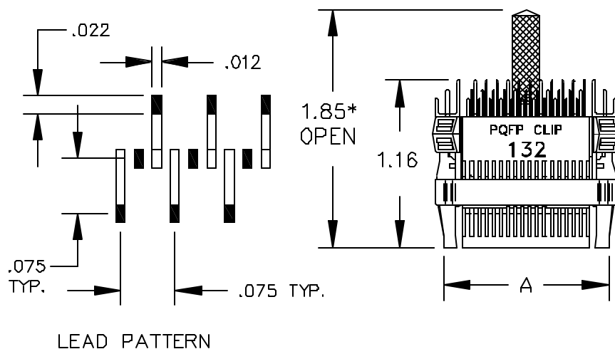
132 PIN JEDEC CHIP
