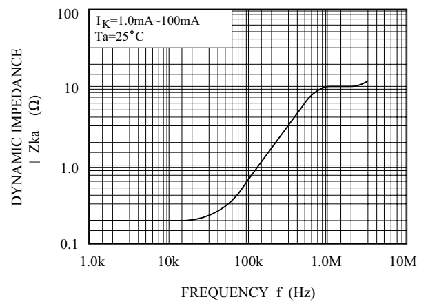
|Z_{ka}| - f
