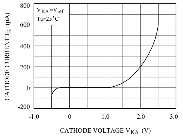
I_K - V_{KA}
