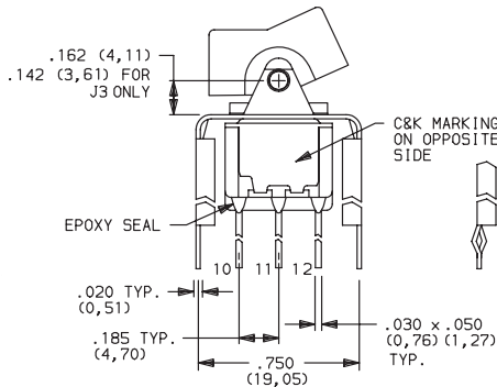
7401J1_BE2 4PDT
