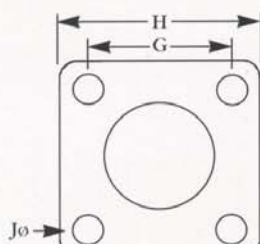
Universal Flange Receptacle
