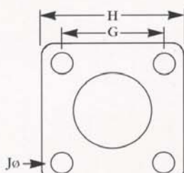
Universal Flange Receptacle
