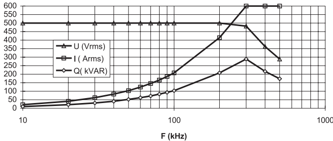
660 nF 500 Vrms FAI16J0664K-- FAI36J0664K--
