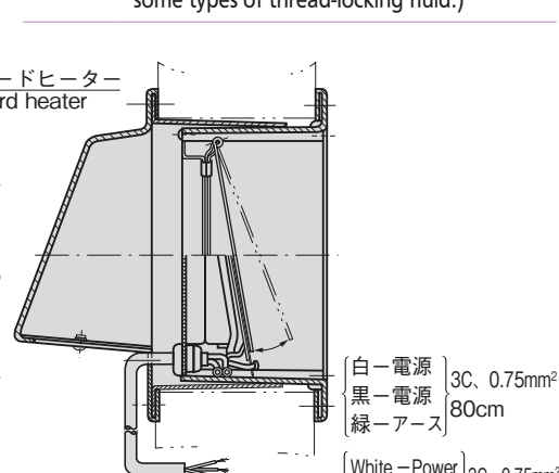
吸気用(A型) Intake(A-type)
