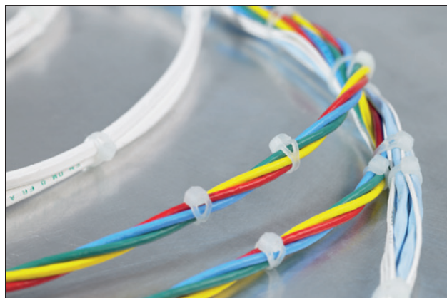
Die gerundete Geometrie der V-Serie bewahrt vor Beschädigung paralleler Kabelstränge.
