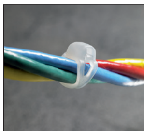
Die V-Serie passt sich sehr gut an Kabelbündel an und hat nur einen geringen Überstand.
