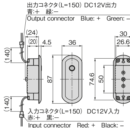
パネル穴明け寸法 Panel drilling dimensions
