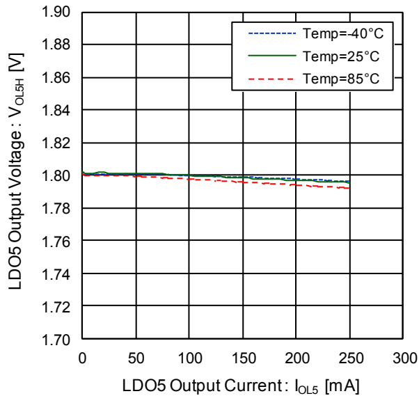
Figure 41. LDO5 Output Voltage vs LDO5 Output Current ( V_{BAT}=3.6\text{V} , V_{SYS}=VIN=VINL1,2 , LDO5VSEL=H)
