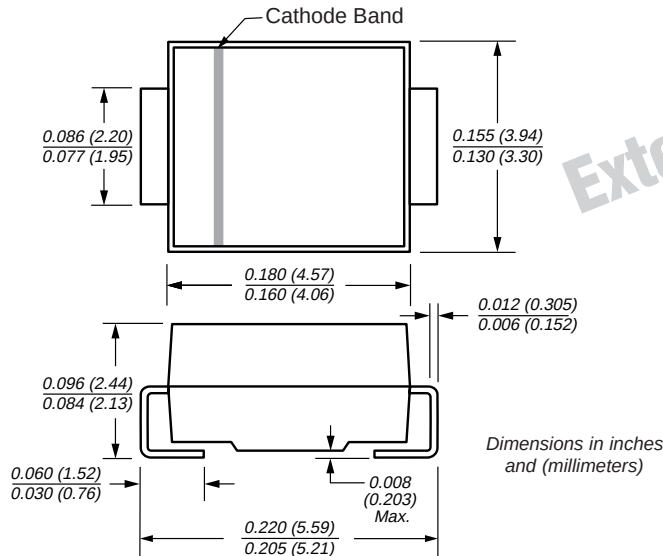
DO-214AA (SMBJ-Bend)
