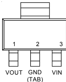
SOT-223
