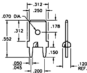
.250 TAB
