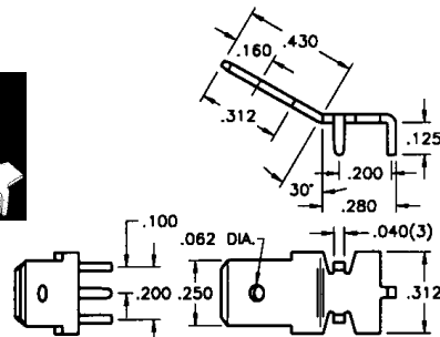
.250 TAB
