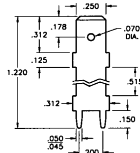
.250 TAB
