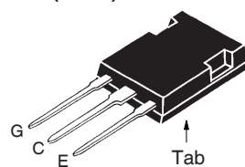
PLUS247 (IXGX)
