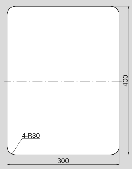
パネル穴明け寸法 Panel drilling dimensions
