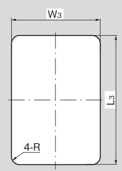
パネル穴明け寸法 Panel drilling dimensions
