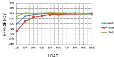
RSD-30H-5
