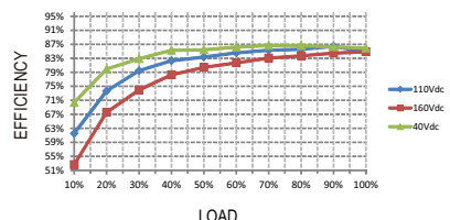
RSD-30H-24
