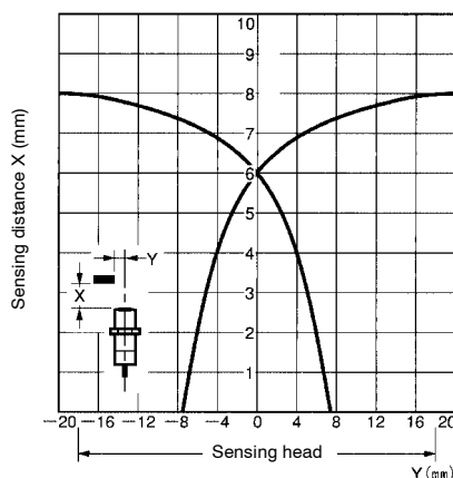
E2ES-X8D1
