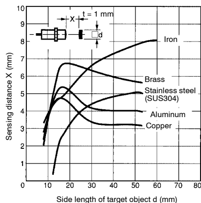
E2ES-X8D1
