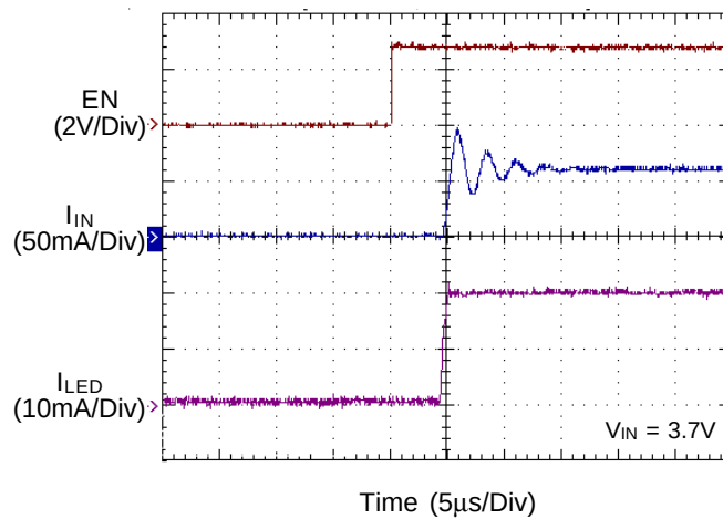
Turn-On
