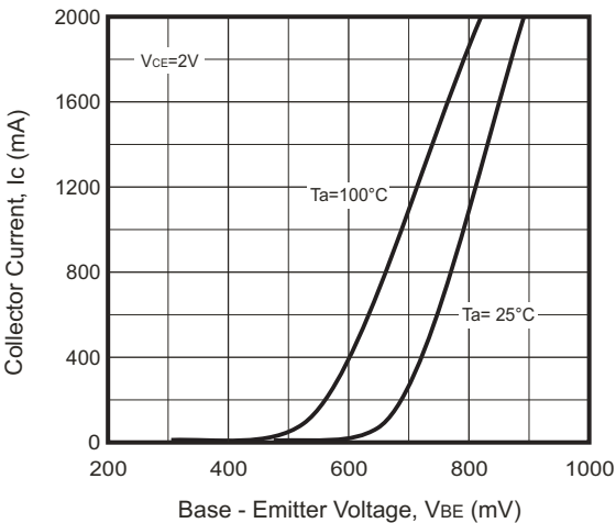
Fig.7 - V_{BE} - I_C
