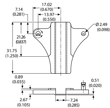
5021NG Ejector
