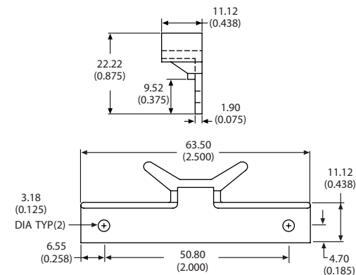
5005-09NG PULLER *
