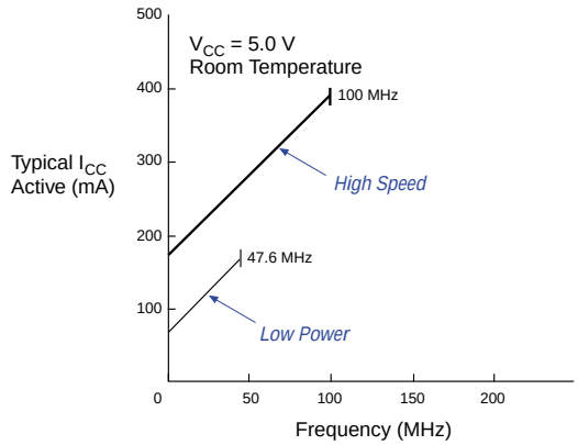
EPM7160E
