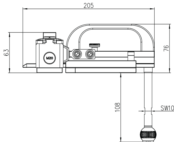
Fig. 8: Türplatte mit Fluchtentriegelung, Abmessungen und Montage/Gate mounting plate with emergency release, measurement and installation/Plaque de porte avec déverrouillage de secours, dimensions et installation
