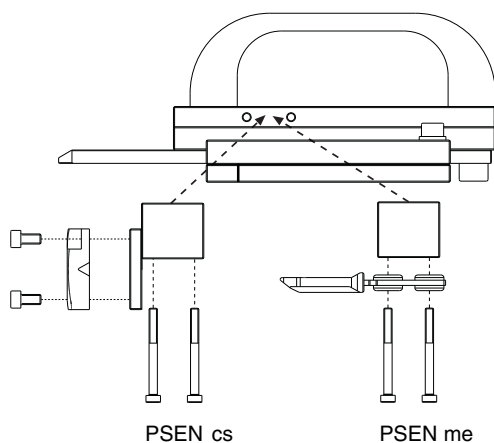
Fig. 4: Betätiger montieren/Install actuator/Montage de l'actionneur
