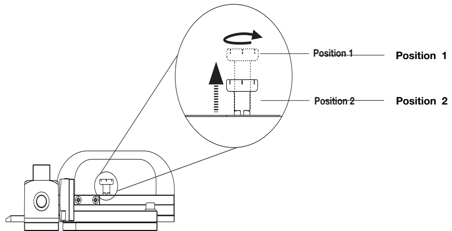
Fig. 3: Türplatte mit Arretierbolzen/Gate mounting plate with locking pin/Plaque de porte avec targette
