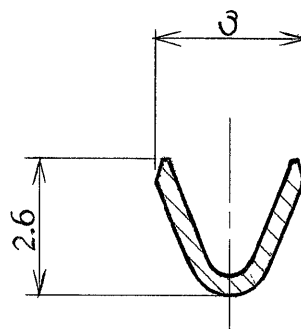
断面 B-B
