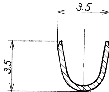
断面 C-C
