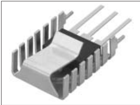
FK 245 MI 247 V 19,7 K/W mit Lötfahne für vertikalen Einbau with solder lug for vertical installation
