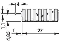
FK 245 MI 247 V 19,7 K/W mit Lötfahne für vertikalen Einbau with solder lug for vertical installation
