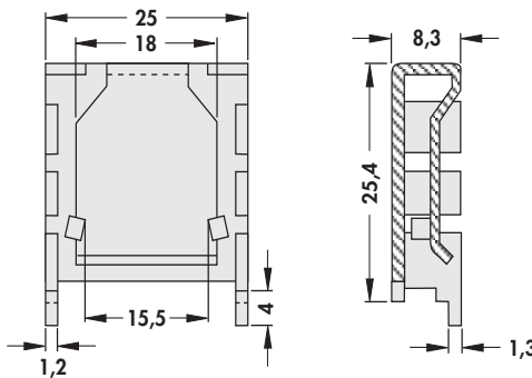
FK 224 SA 218 1 FK 224 MI 218 1
