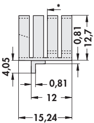
FK 242 SA 220 H 26 K/W
