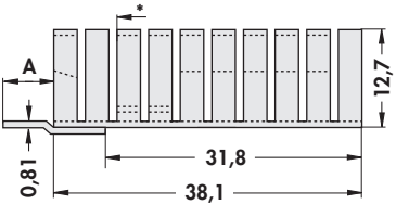
FK 240 SA 220... 16 K/W
