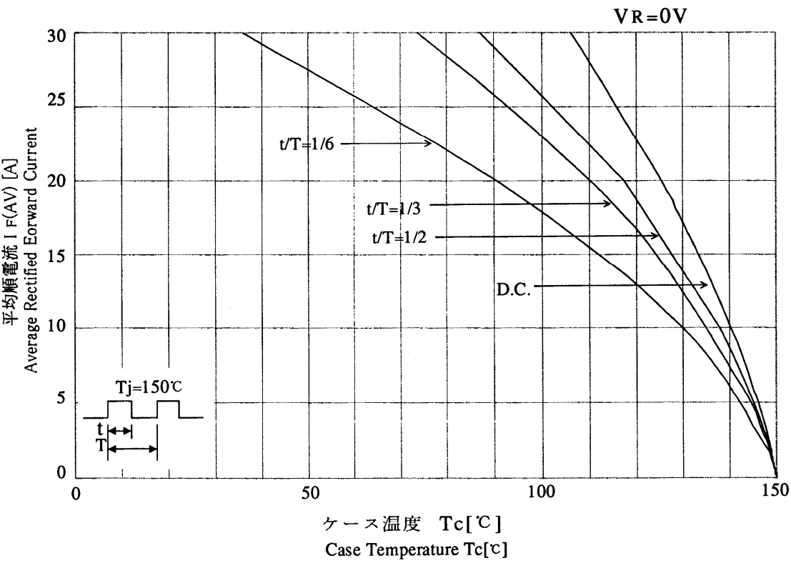
T_c - I_{F(AV)} 特性 Characteristics
