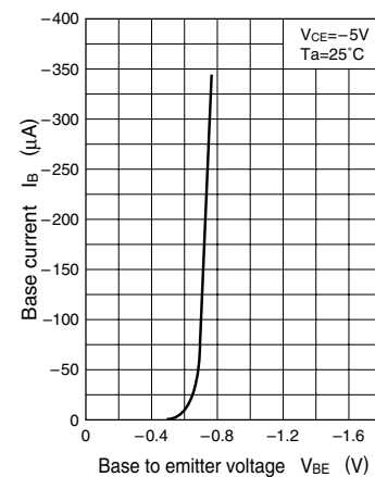
I_B - V_{BE}
