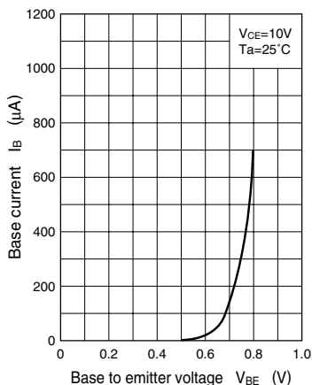
NV - I_C
