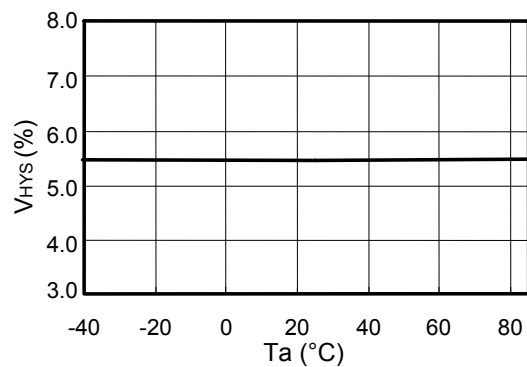
S-80860CL
