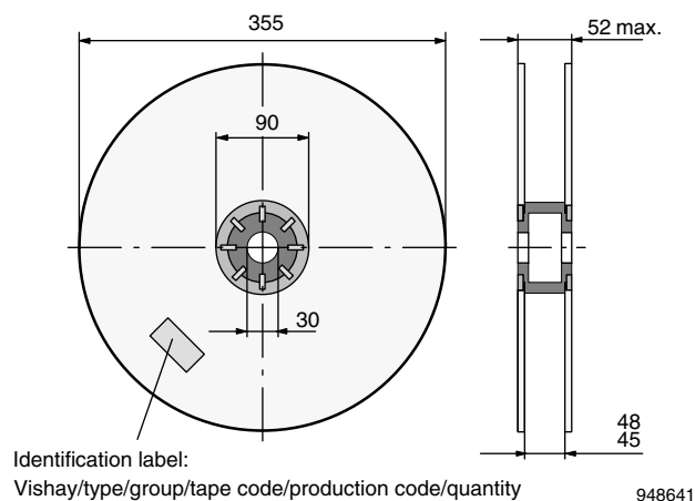
Fig. 18 - Reel
