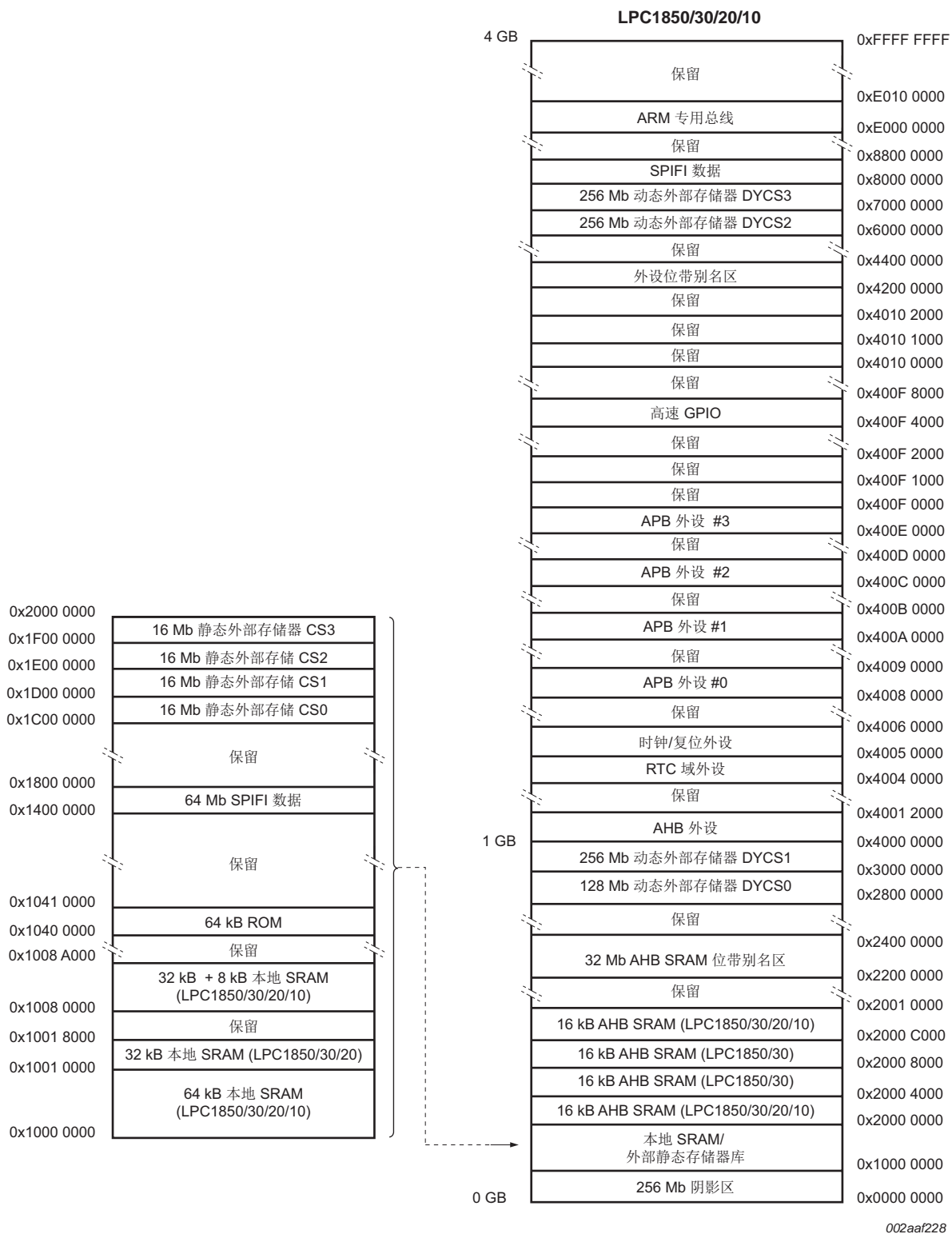
图 9. LPC1850/30/20/10 存储器映射 (概述)
