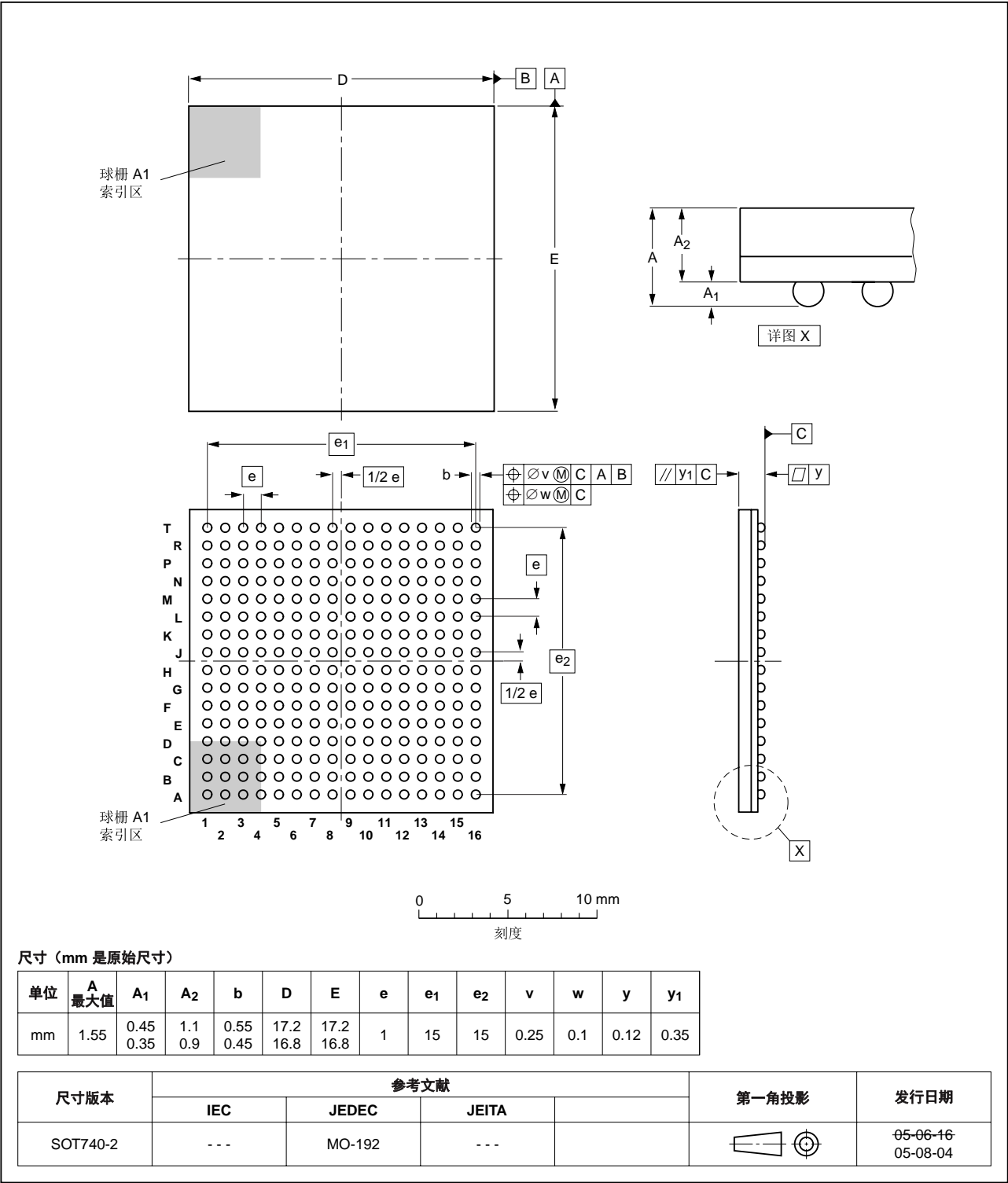
图 41. LBGA256 封装的封装尺寸
