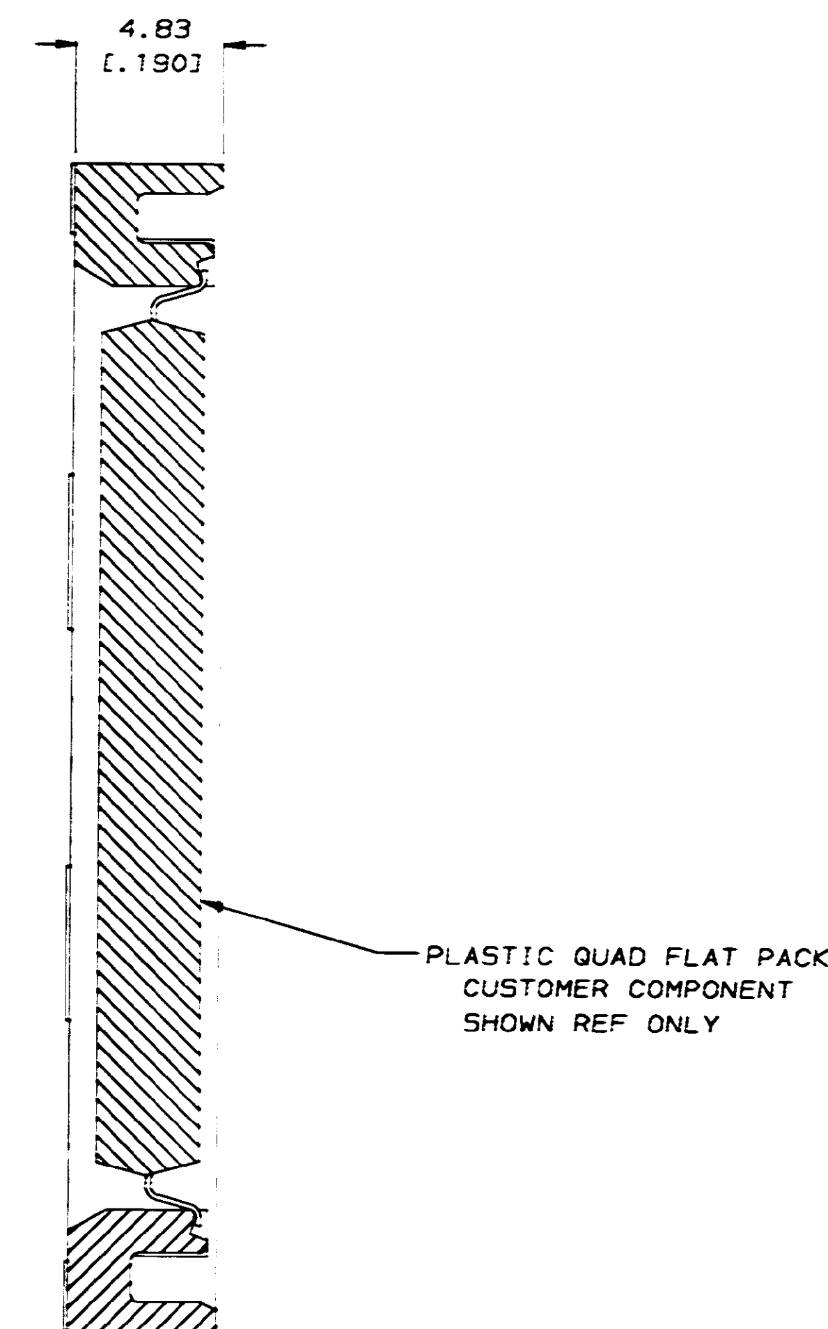
SECTION A-A
