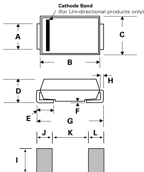
DO-214AA (SMB J-Bend)
