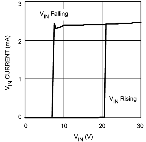
VIN UVLO
